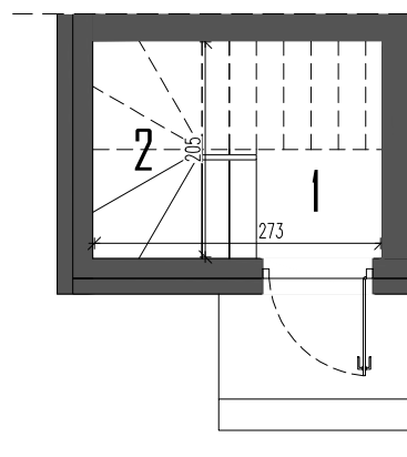
RZUT PARTERU
