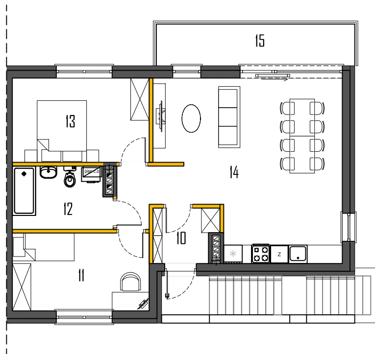
RZUT PIĘTRA
