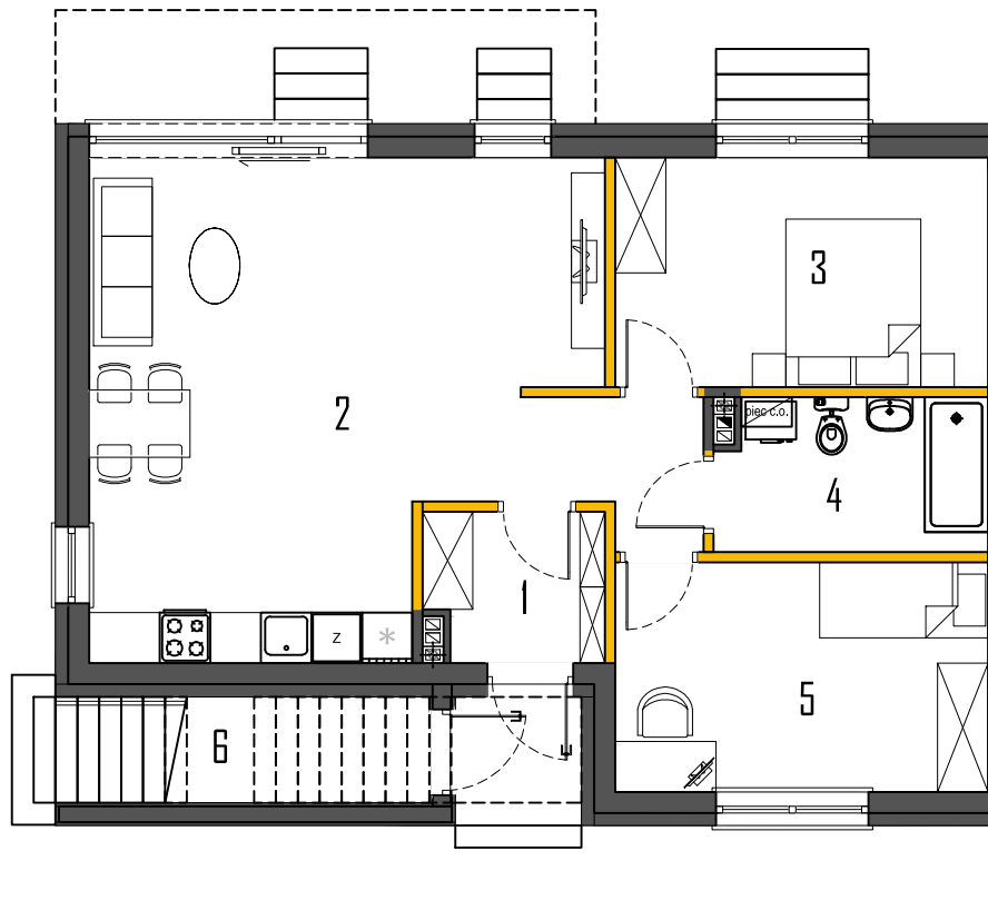
RZUT PARTERU
