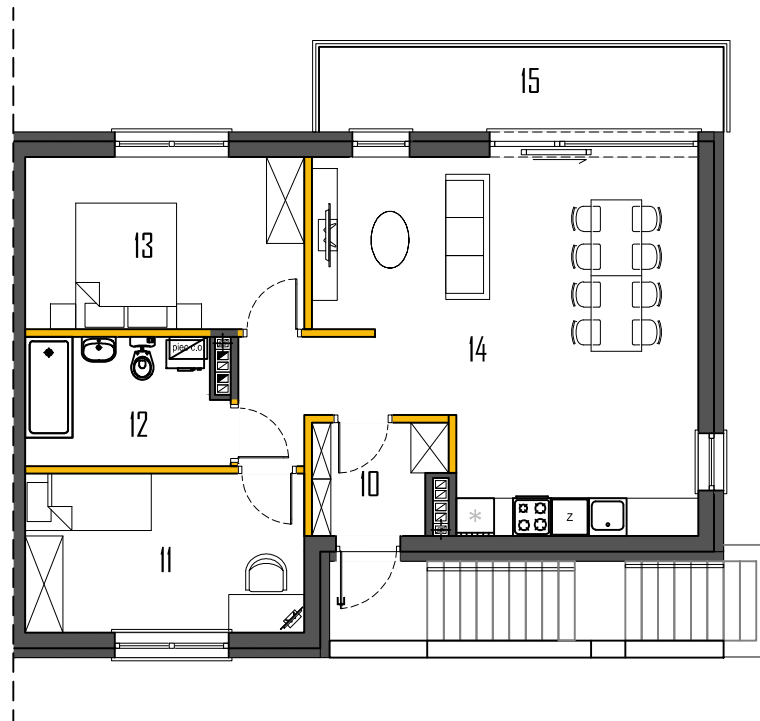
RZUT PIĘTRA
