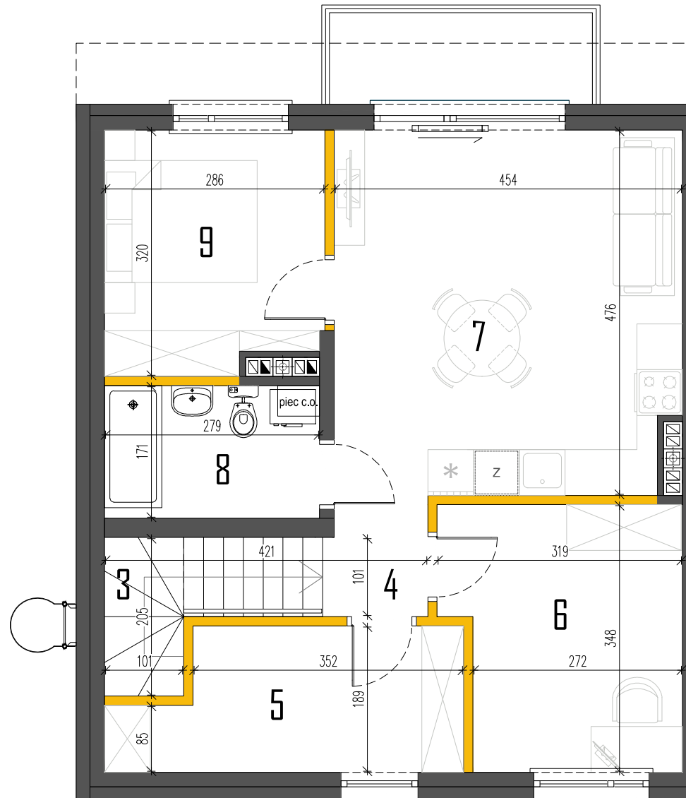
RZUT PIĘTRA
